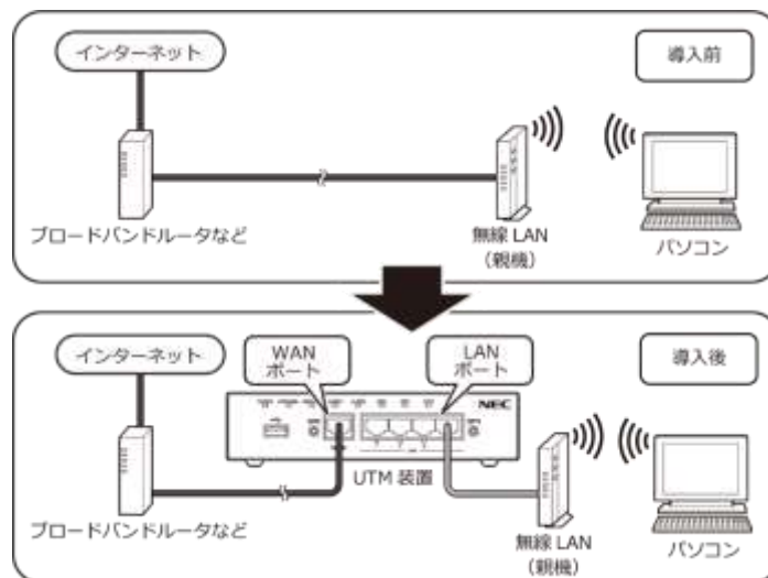
図 3-5 ブロードバンドルータなどの配下に無線 LAN（親機）を使用している場合の UTM 接続位置
