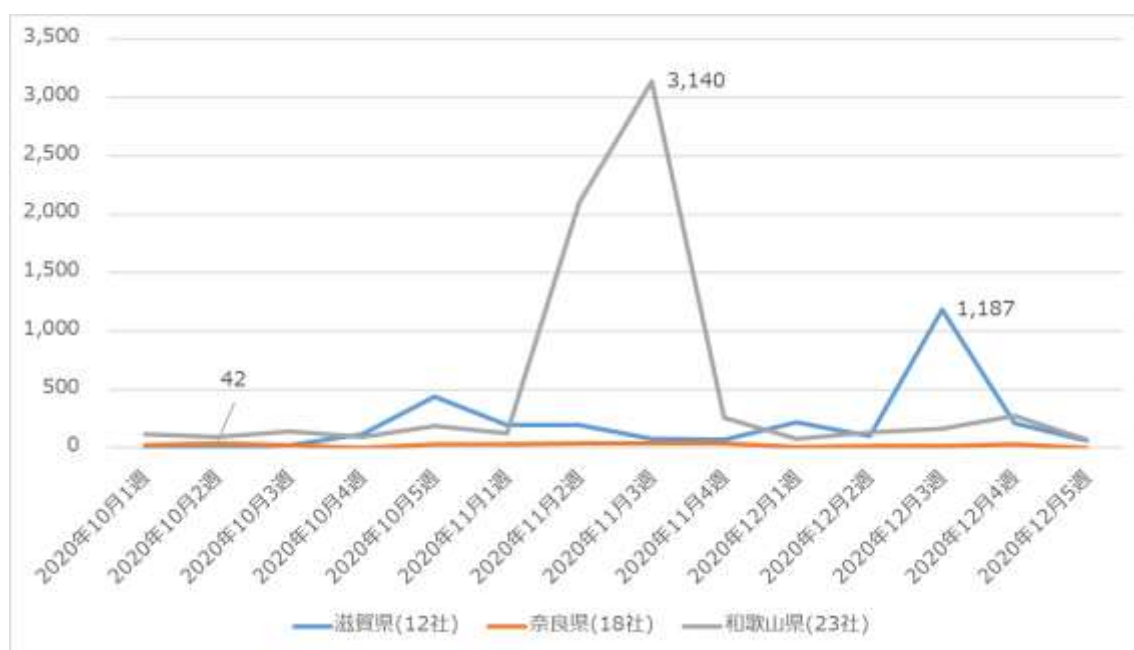
図 4-23 UTM 脅威検知数の推移 (IPS) (所在地別)
