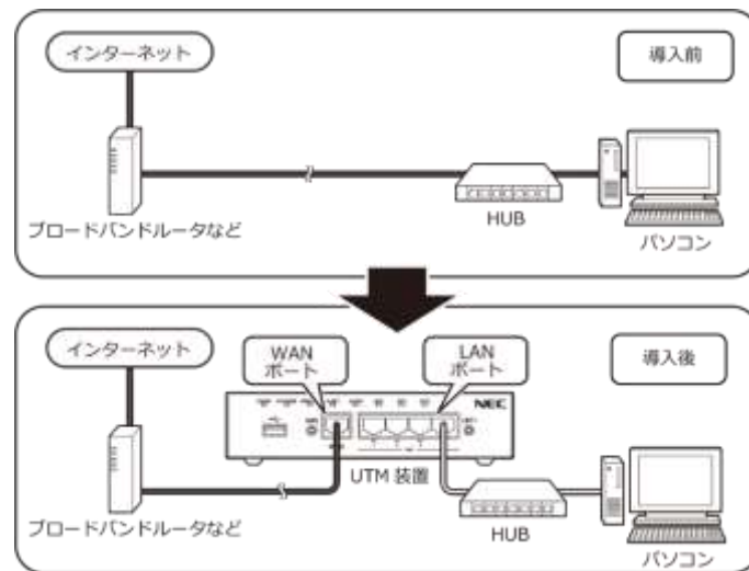
図 3-4 ブロードバンドルータなどの配下に HUB などを設置している場合の UTM 接続位置
